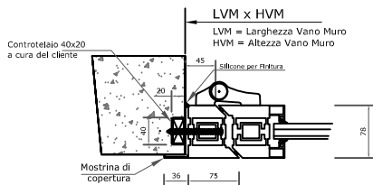
MONTAGGIO A SPIGOLO
