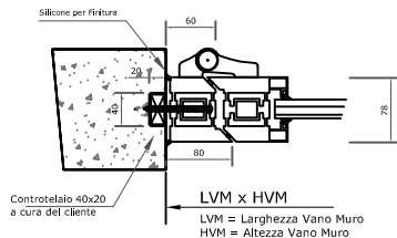
MONTAGGIO A CORRIDOIO
