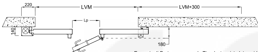
Esempio di Portone scorrevole Tira destro vista lato guida con porta pedonale verso a Tirare DX
