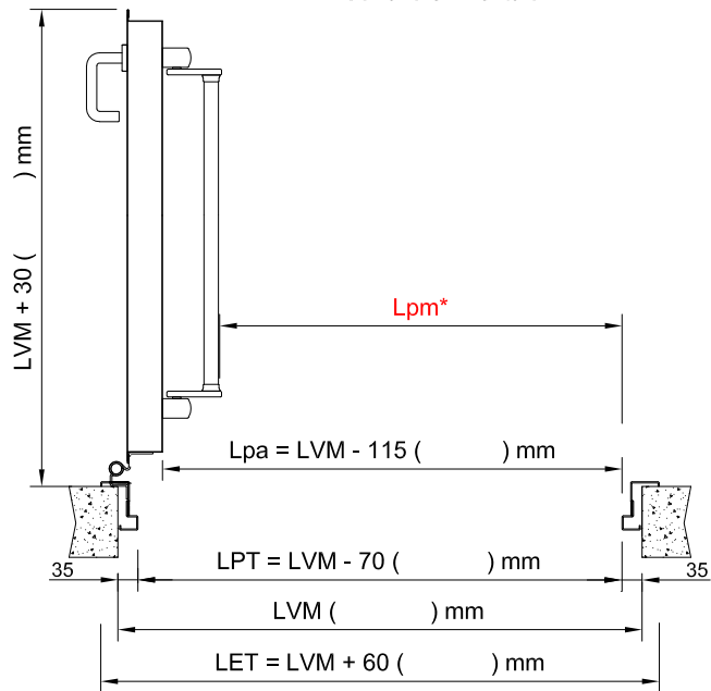
Sezione Orizzontale
