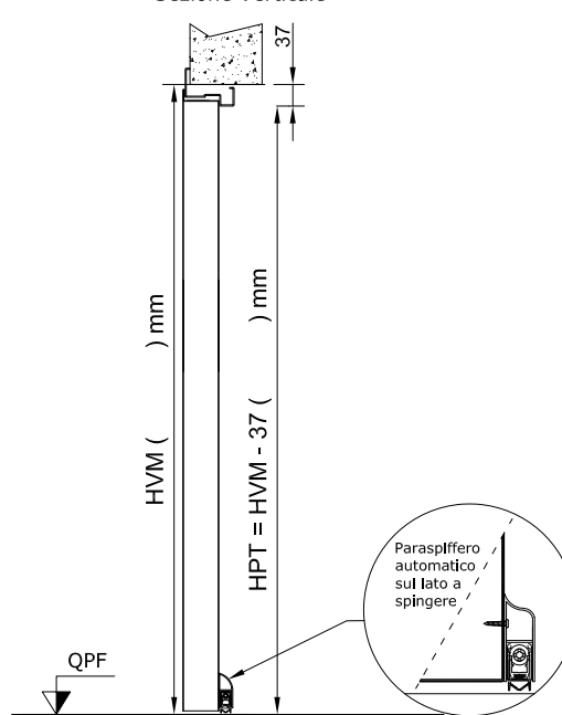
Sezione Verticale
